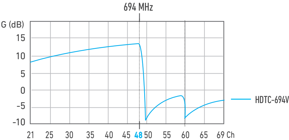
Diagrama de ganancia
